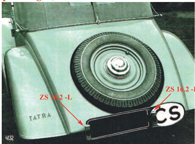
Tatra 75 - příklad umístění ZS 16 na vozidle,- ZS 16 - Lampen am Wagen
