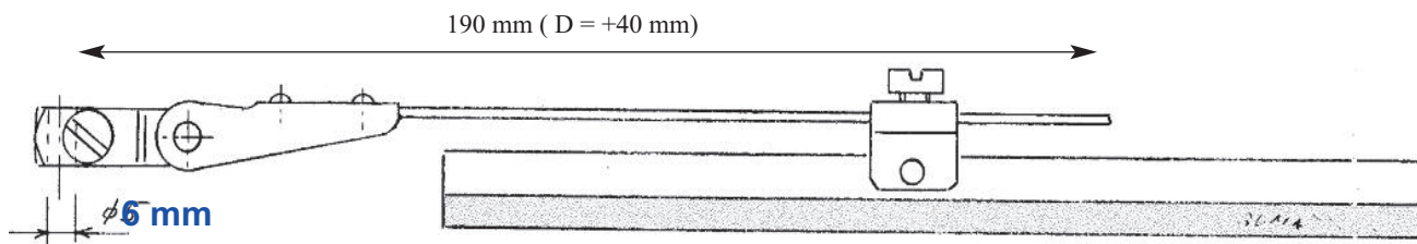
RS -1-6mm Kč 2230,- Raménko stěrače úplněchromované ; RS -1D-6mm Kč 2480 Raménko stěrač úplněchromované ; Kompletter Wischerarm verchromt ; Kompletter Wischerarm verchromt Arm of wiper complete chromed plated ; Arm of wiper complete chromed plated
