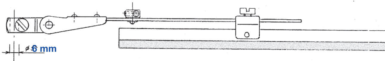
RS-3 - 6mm Kč 2515,- Raménko stěrače s kloubem propojky Wischerarm mit Verbindungsgelenk Arm of wiper with joint-interkonektion
